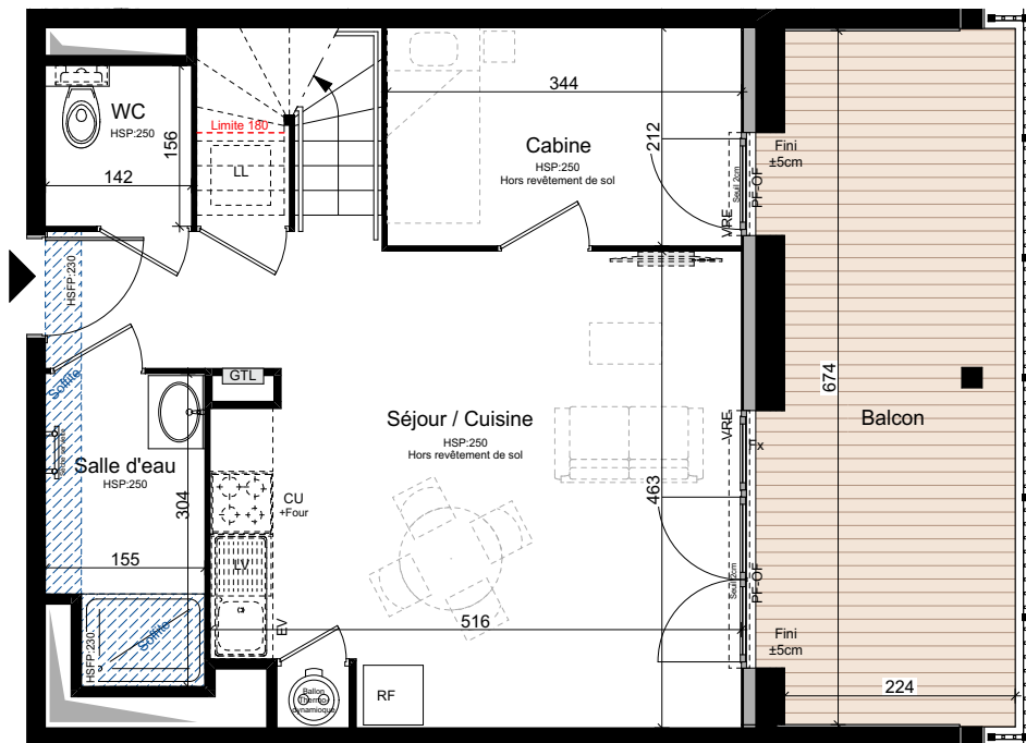
Niveau R+2
