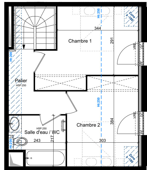
Niveau Combles
